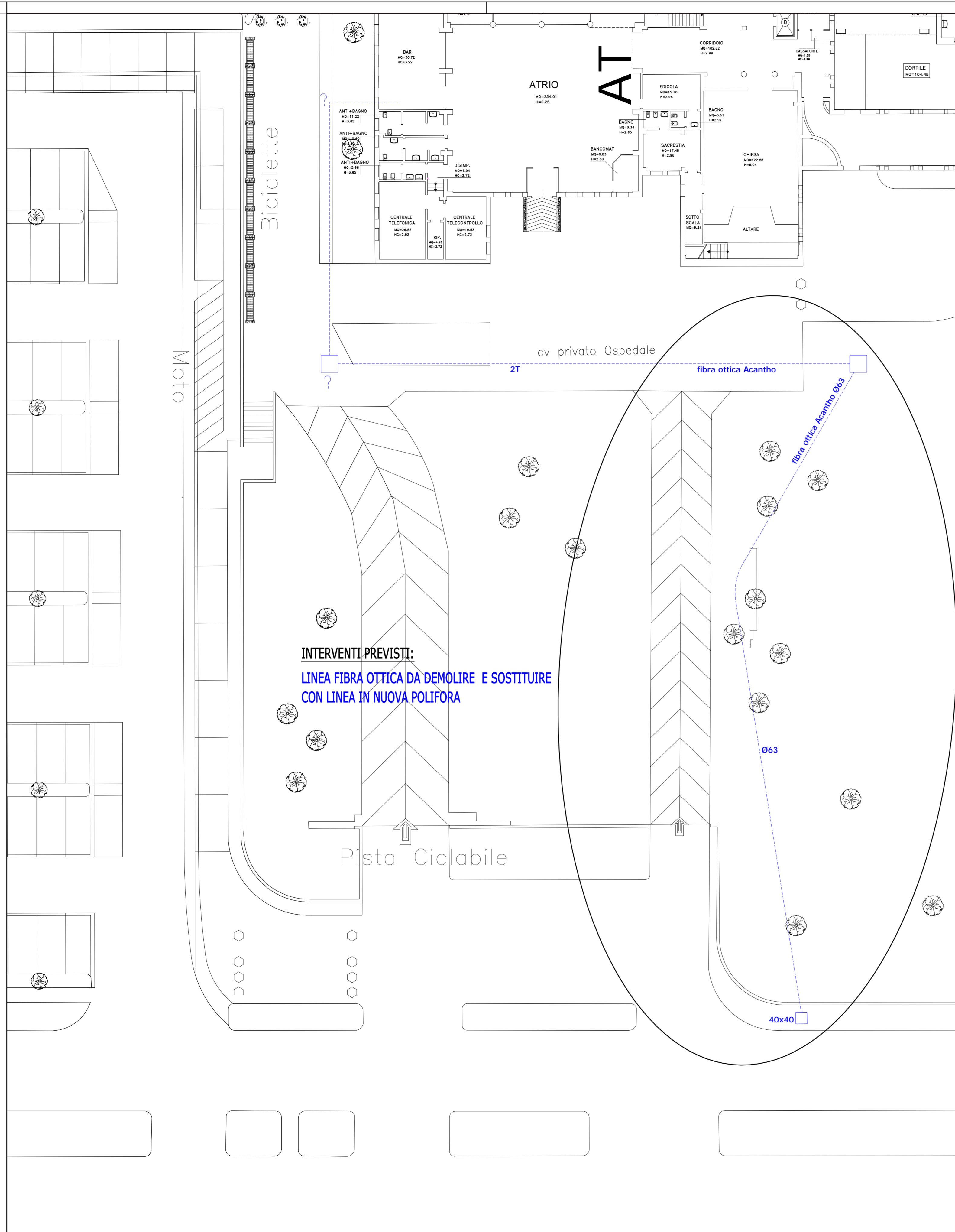
SITUAZIONE ESISTENTE PIANO TERRA - SCALA 1:200
