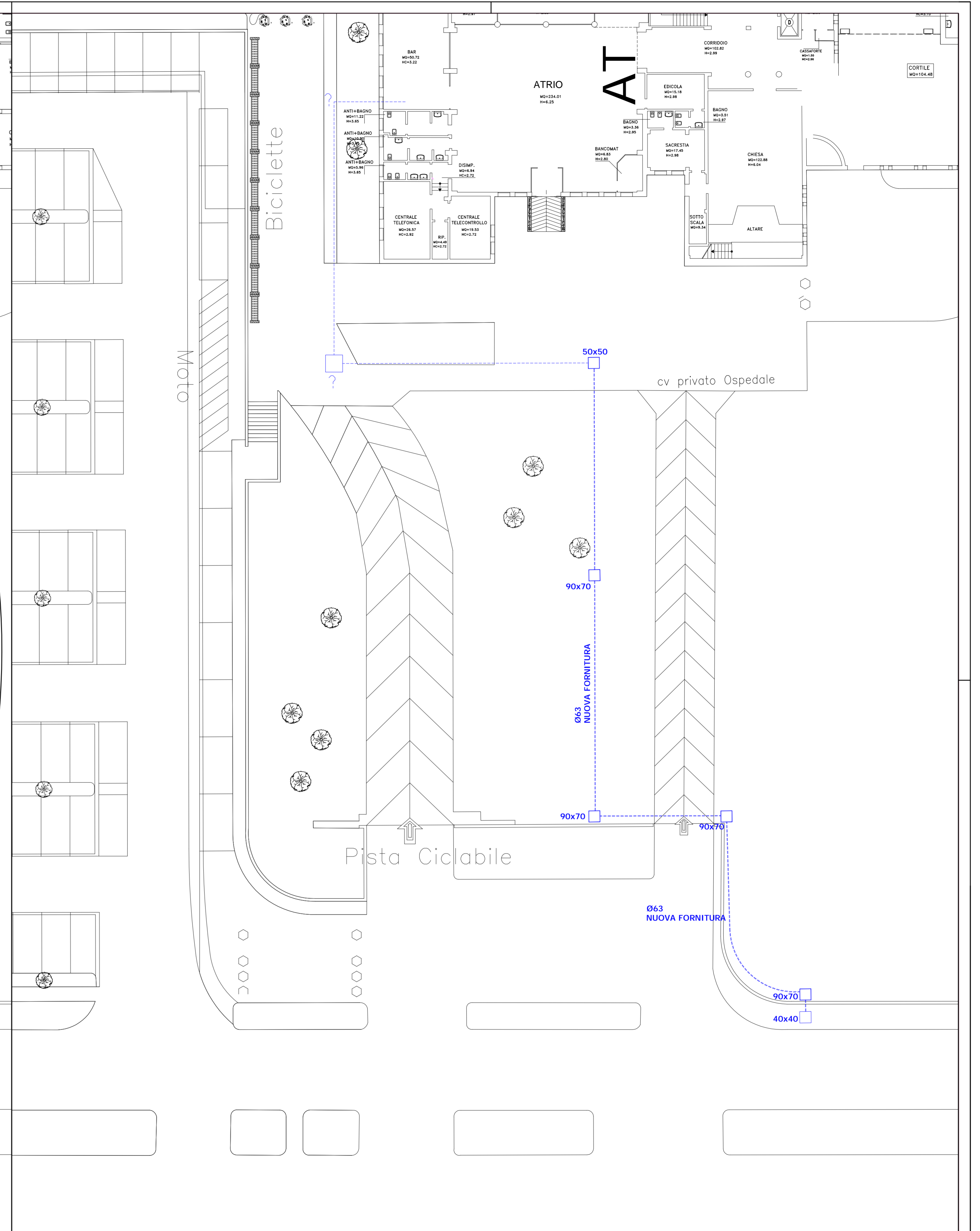
SITUAZIONE DI PROGETTO PIANO TERRA - SCALA 1:200
